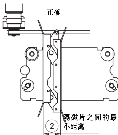
关门门刀系统
